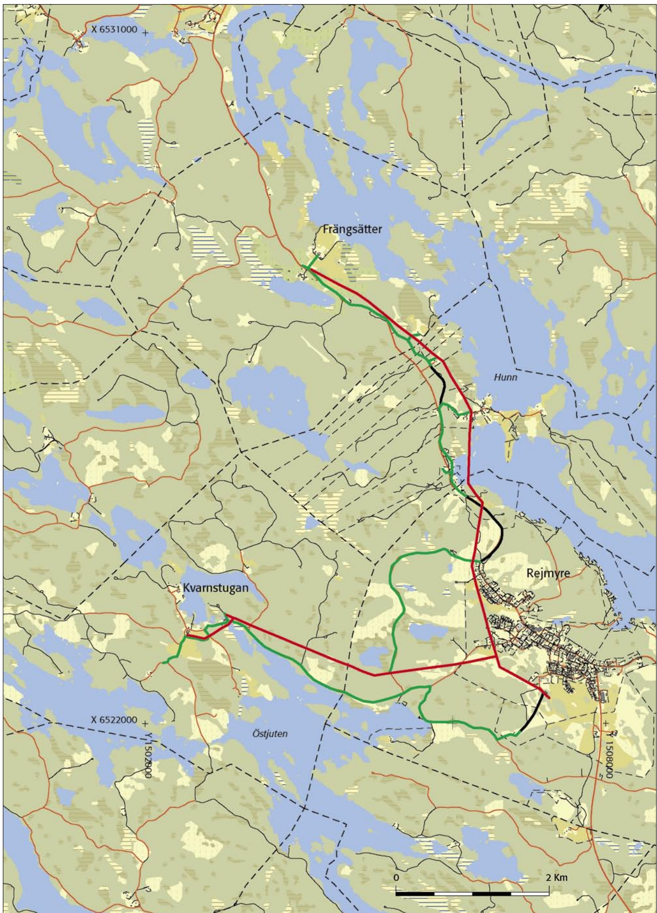
Fig 2. Utdrag ur Fastighetskartan (9G 5a, 9G 5b, 9G 4a, 9G4b), skala 1:50 000. De större sjöarna och några orter utsatta. Grön linje representerar ursprunglig sträckning för jordkabelnedläggning. Svart linje representerar ändring av kabelnedläggning. Röd linje representerar sträckning för luftledningsrasering.
